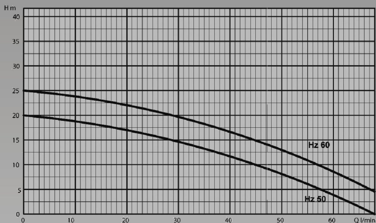
Teljesítménydiagram
