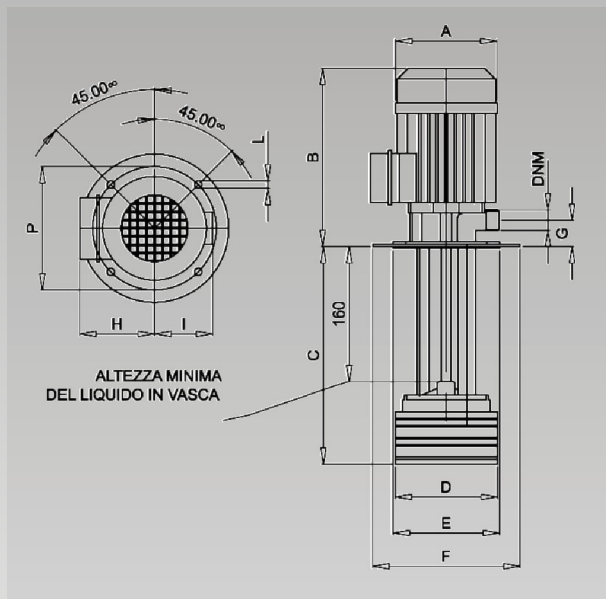
Beépítési méretek
