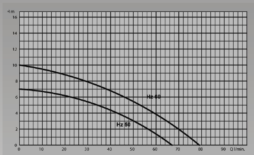
Teljesítménydiagram
