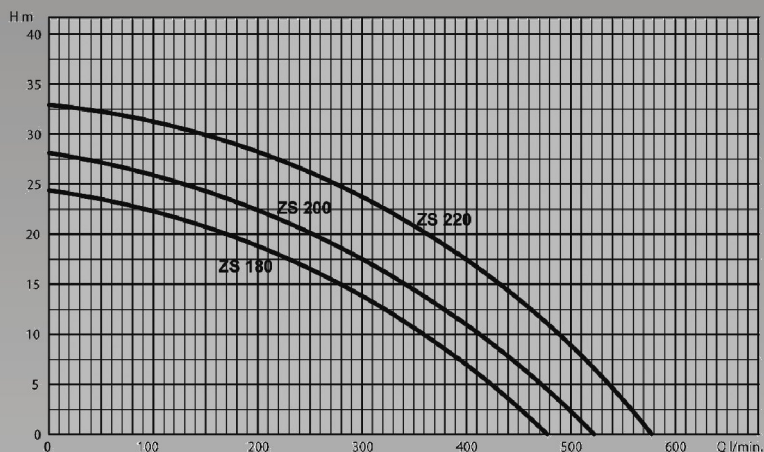
Teljesítménydiagram
