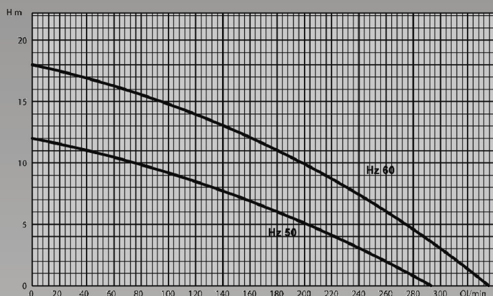
Teljesítménydiagram
