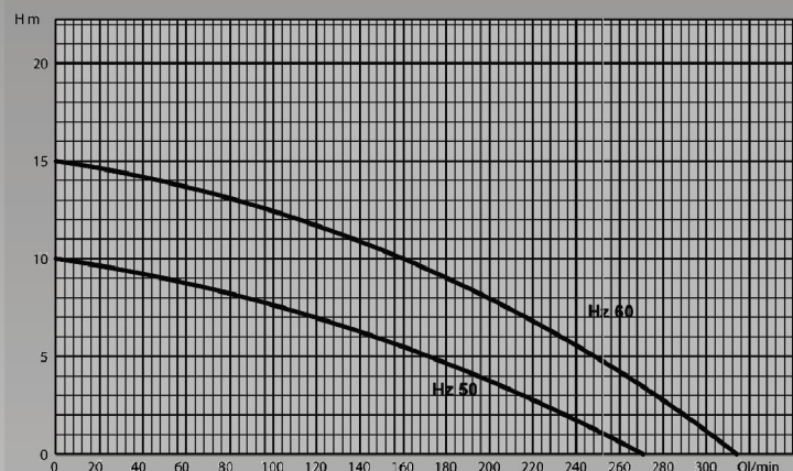
Teljesítménydiagram
